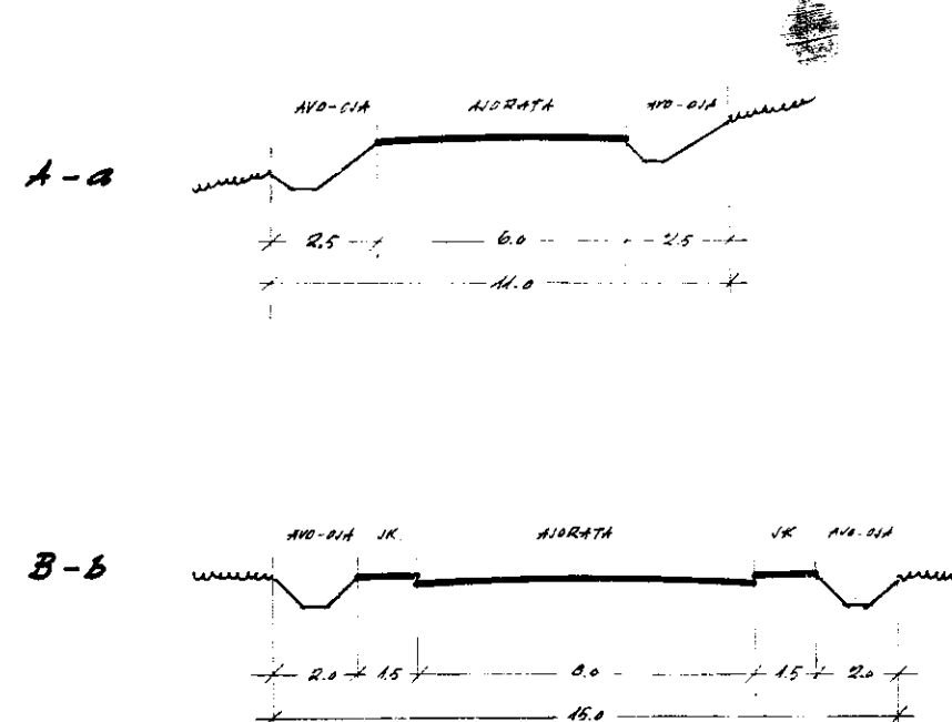
KATUJEN POIKKILEIKKAUKSET 1:200
